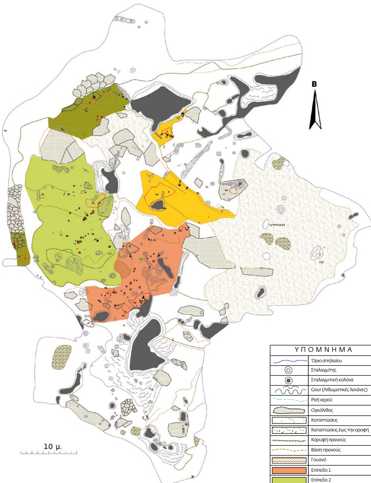
02 Οριζοντιογραφία του σπηλαίου Ανδρίτσας. Κάθε επίπεδο αποδίδεται με διαφορετικό χρώμα. Τοπογραφική αποτύπωση: Θεόδωρος Χατζηθεοδώρου, Ευθυμία Τσάκου.
