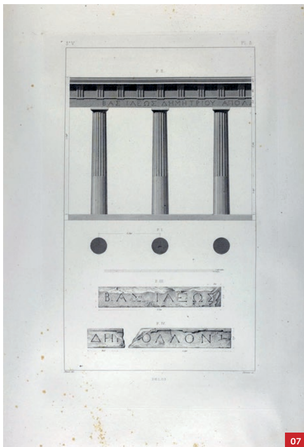
07 Σχεδιαστικές αποτυπώσεις στοιχείων της ζωφόρου της Στοάς του Φιλίππου Ε΄ με την αφιερωματική επιγραφή του μνημείου και αποκατάσταση τμήματος της κιονοστοιχίας του — σε όψη και σε κάτοψη— από τον Α. Blouet ( Expédition scientifique de Morée III , Παρίσι 1838, πίν. V).
