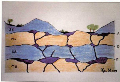
1. Σχηματική στρωματογραφία του υπεδρόρου της Λαυρεωτικής. Α, Β, Γ: Πρώτη, Δεύτερη και Τρίτη Μεταλλοφόρος Επαφή, αντίστοιχα. Σ1: Ανώτερος Σχιστόλιθος, Μ1: Ανώτερο Μάρμαρο Σ2: Κατώτερος Σχιστόλιθος, Μ2: Κατώτερο Μάρμαρο. Το ιώδες χρώμα δηλώνει τα μεταλλοφόρα κοιτάσματα.
