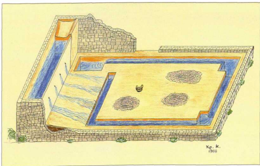
2. Σχηματική παράσταση Ορθογωνίου πλυντηρίου μεταλλεύματος Τύπου Ι.
