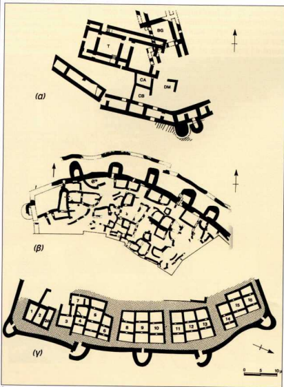
9. Οχυρώσεις των προϊστορικών χρόνων: α. Λέρνα (2650-2100) β. Καστρί Σύρου (2300-2100) γ. Κολώνα Αίγινας (2200-2050).
