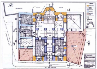
6. Αποτύπωση, κάτοψη ισόγειου.
