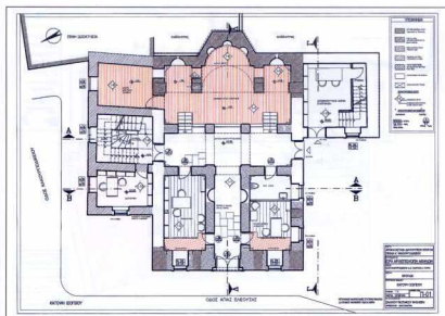
9. Πρόταση, κάτοψη ισόγειου.
