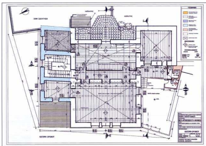
7. Αποτύπωση, κάτοψη ορόφου.
