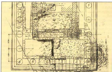
Σχέδιο ανατολικού περασίου-πρόδρομου. Υπολογισμός μεταξονίων.
