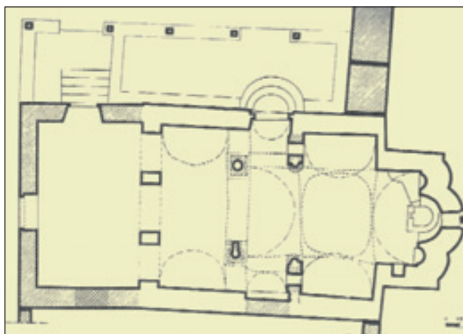
6. Παναγία Κορακονησίας. Κάτοψη.
